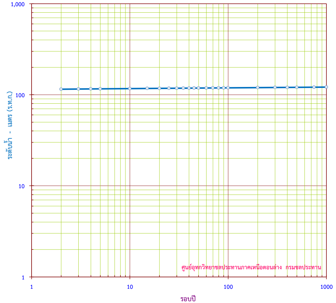
กราฟแสดง ระดับน้ำสูงสุดรายปี ขนาดรอบปีต่างๆ สถานี S.4B อ.เมือง จ.เพชรบูรณ์
