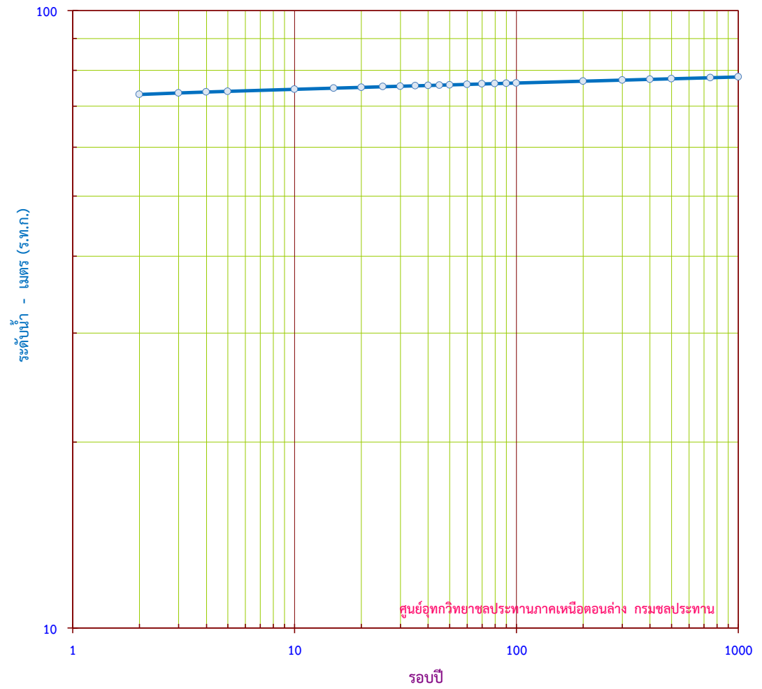
กราฟแสดง ระดับน้ำสูงสุดรายปี ขนาดรอบปีต่างๆ สถานี N.12A บ.หาดไม้ อ.ท่าปลา จ.อุตรดิตถ์
