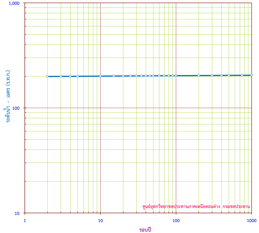
กราฟแสดง ระดับน้ำสูงสุดรายปี ขนาดรอบปีต่างๆ สถานี N.36 บ.หนองกระท้าว อ.นครไทย จ.พิษณุโลก
