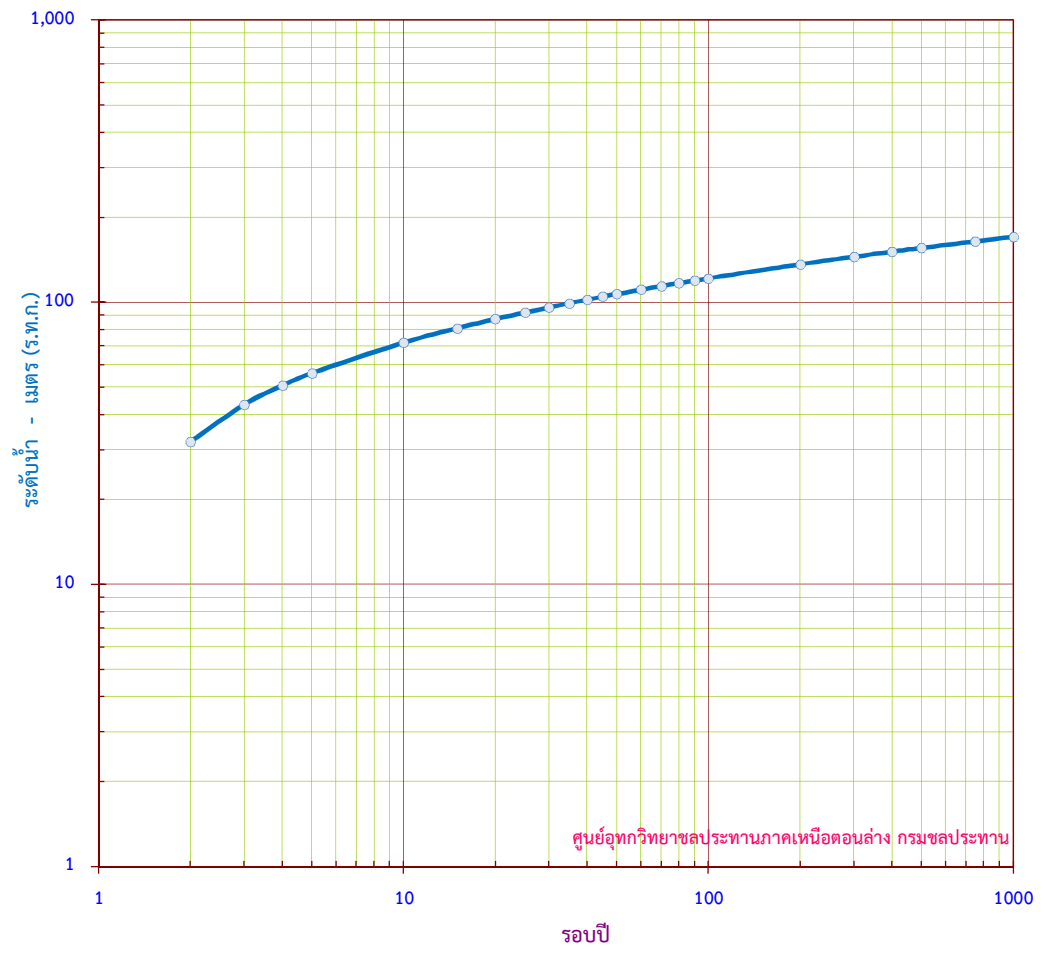
กราฟแสดง ระดับน้ำสูงสุดรายปี ขนาดรอบปีต่างๆ สถานี N.40 บ.หนองบอน อ.วัดโบสถ์ จ.พิษณุโลก
