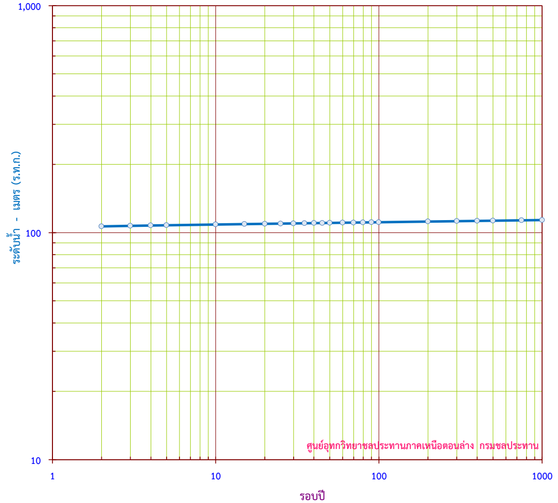
กราฟแสดง ระดับน้ำสูงสุดรายปี ขนาดรอบปีต่างๆ สถานี N.54 บ.วังโป่ง อ.วังโป่ง จ.เพชรบูรณ์
