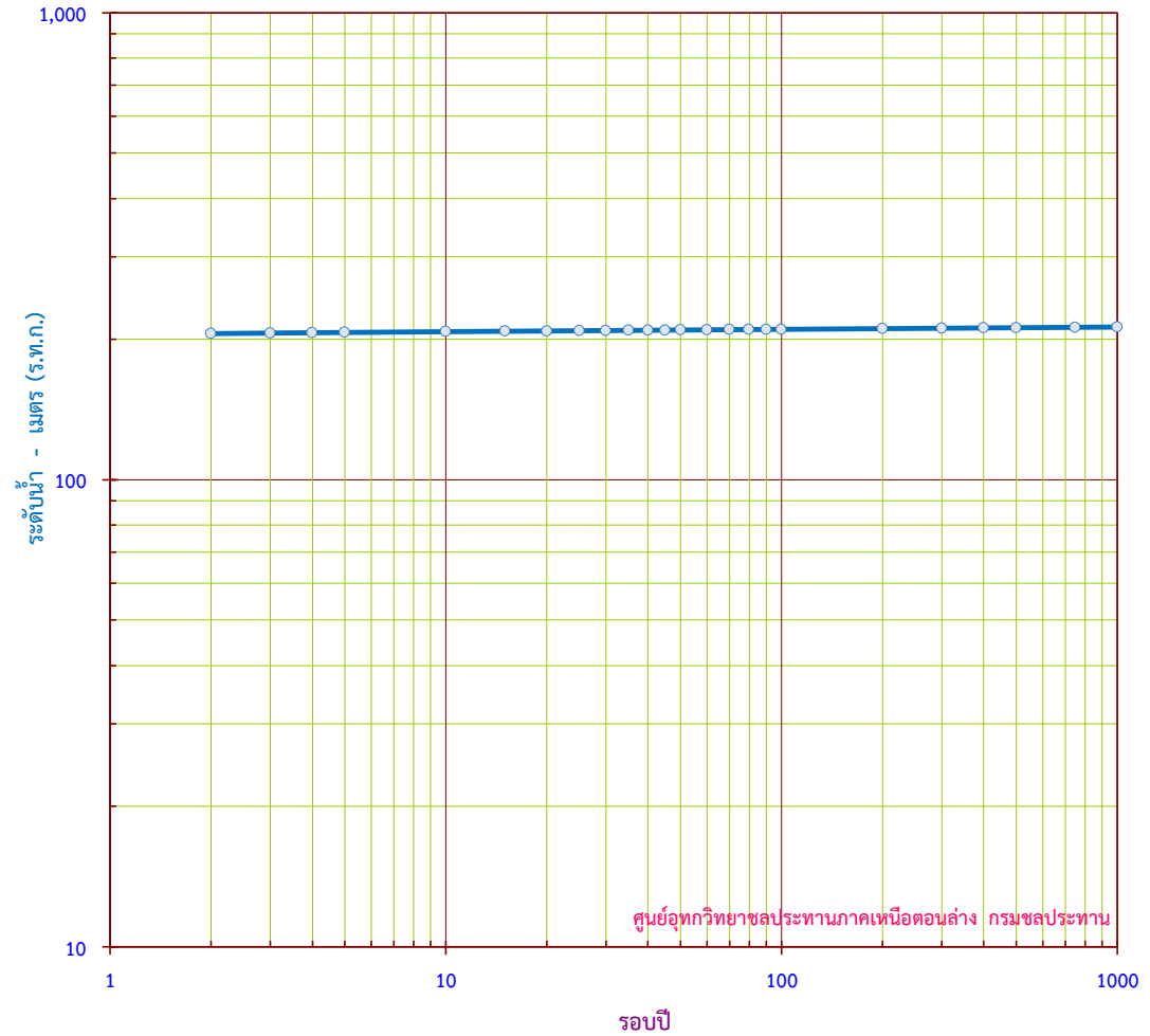
กราฟแสดง ระดับน้ำสูงสุดรายปี ขนาดรอบปีต่างๆ สถานี N.59 บ.นาโพธิ์นาจวน อ.นครไทย จ.พิษณุโลก
