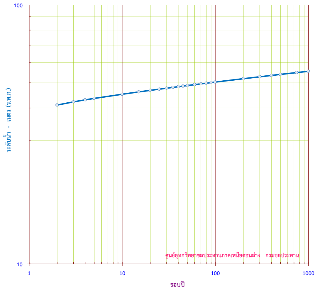
กราฟแสดง ระดับน้ำสูงสุดรายปี ขนาดรอบปีต่างๆ สถานี N.5A ในเมือง อ.เมือง จ.พิษณุโลก
