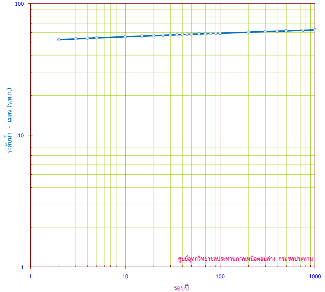
กราฟแสดง ระดับน้ำสูงสุดรายปี ขนาดรอบปีต่างๆ สถานี N.60 บ.เด่นสำโรง อ.ตรอน จ.อุดรดิตถ์
