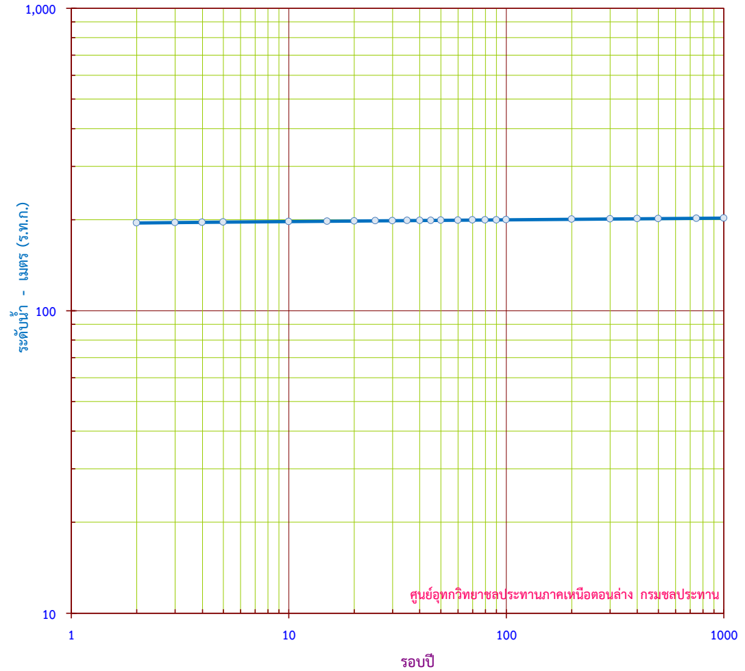
กราฟแสดง ระดับน้ำสูงสุดรายปี ขนาดรอบปีต่างๆ สถานี N.62 บ.ห้วยท่าเนื้อ อ.ชาติตระการ จ.พิษณุโลก
