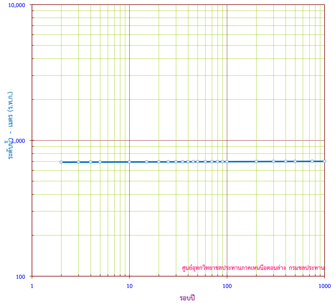
กราฟแสดง ระดับน้ำสูงสุดรายปี ขนาดรอบปีต่างๆ สถานี N.73 บ.ทานตะวัน อ.เข็กน้อย จ.เพชรบูรณ์
