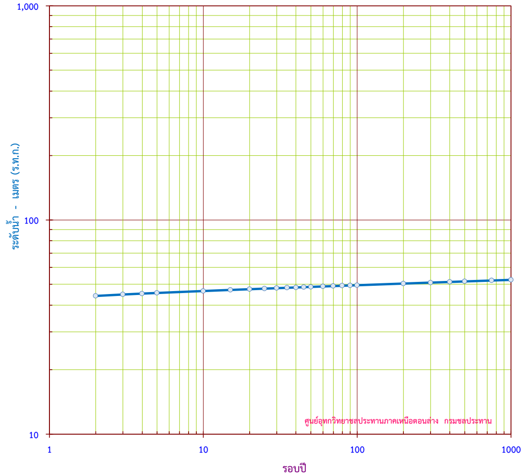
กราฟแสดง ระดับน้ำสูงสุดรายปี ขนาดรอบปีต่างๆ สถานี P.16 อ.ชาณุวรลักษบุรี จ.กำแพงเพชร
