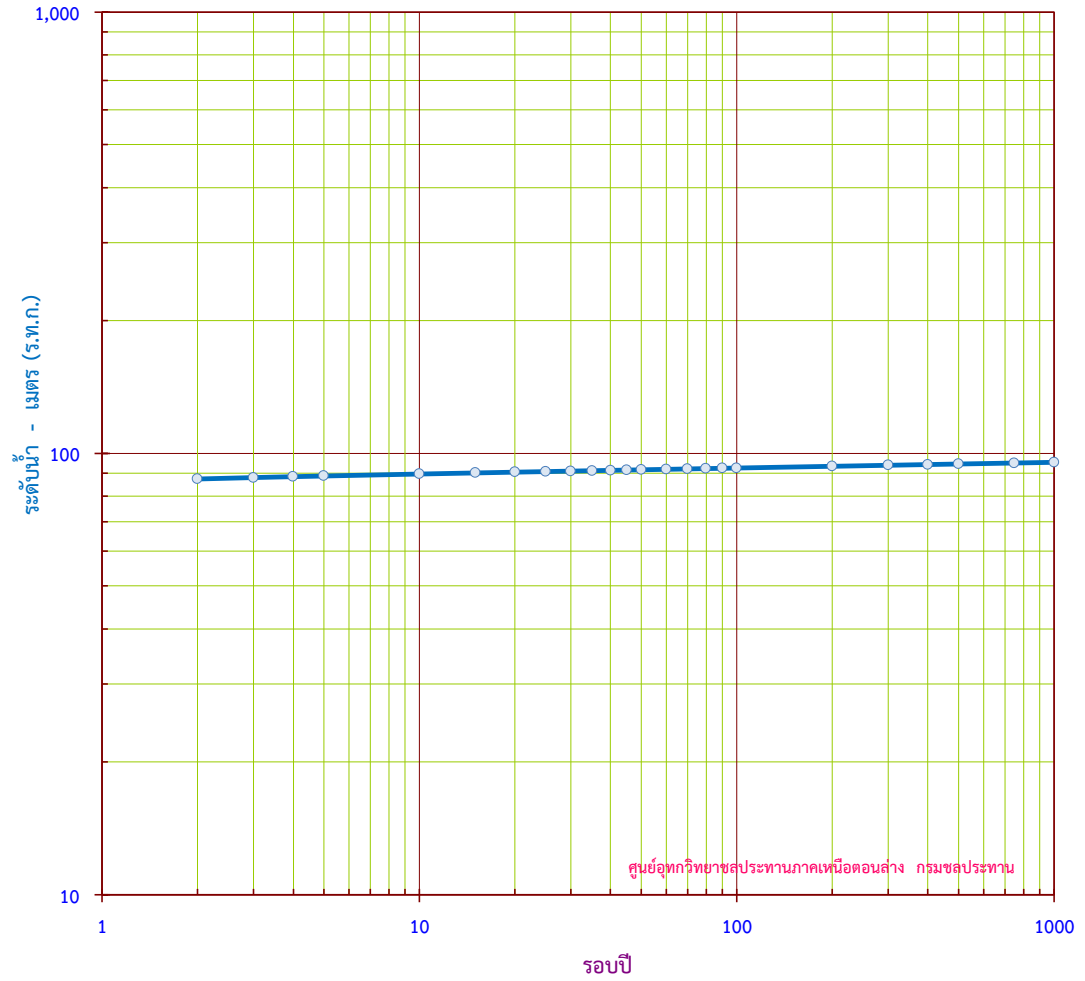
กราฟแสดง ระดับน้ำสูงสุดรายปี ขนาดรอบปีต่างๆ สถานี P.26A อ.เมือง จ.กำแพงเพชร
