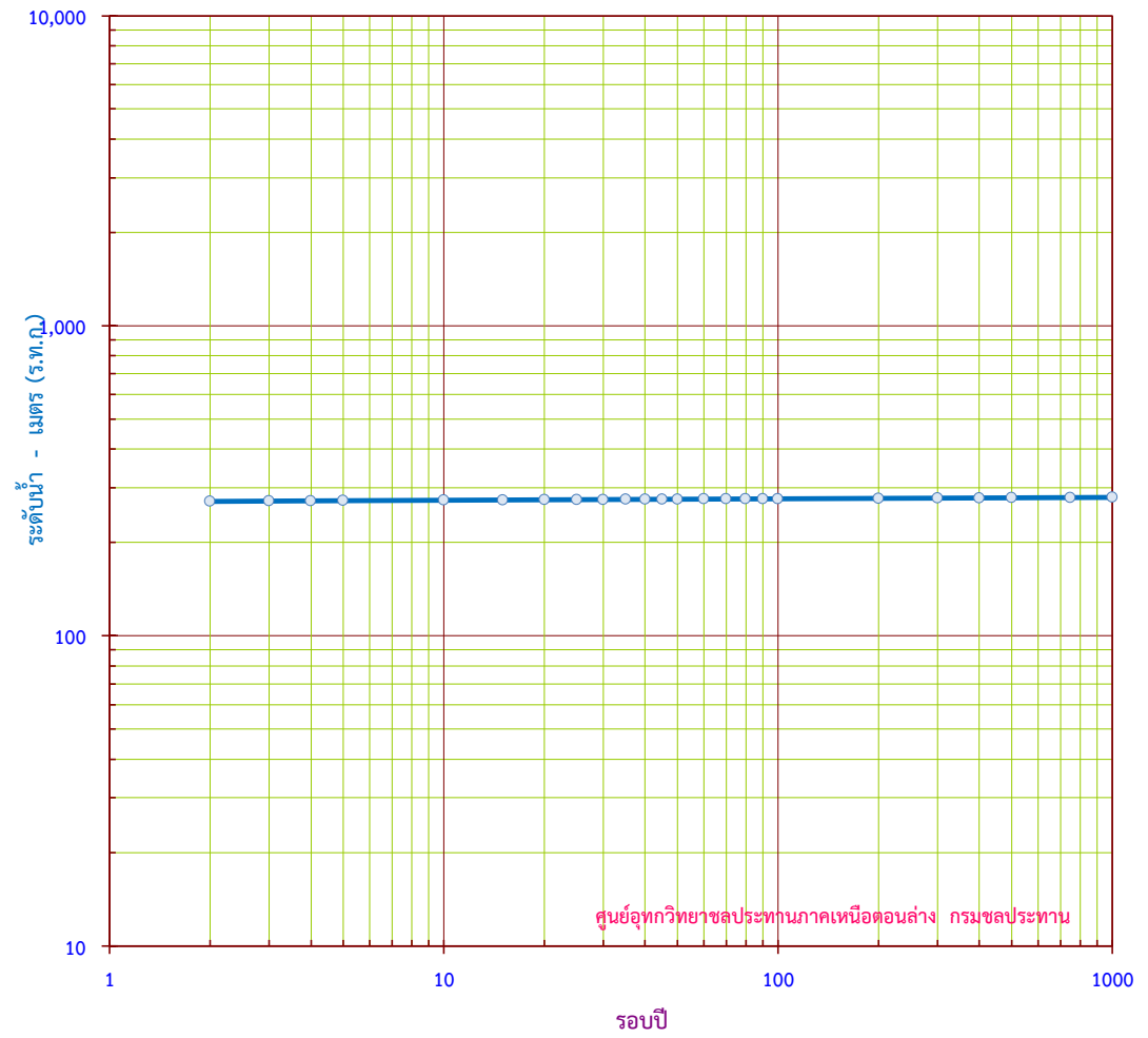
กราฟแสดง ระดับน้ำสูงสุดรายปี ขนาดรอบปีต่างๆ สถานี SW.6 อ.แม่สอด จ.ตาก
