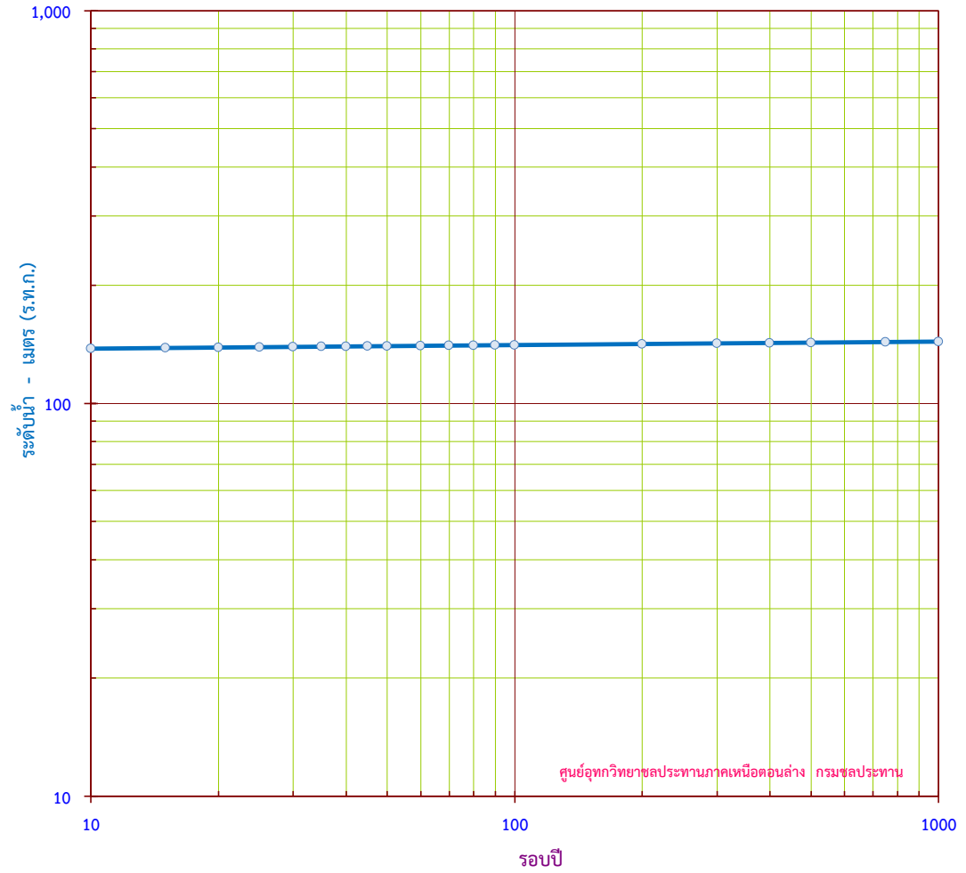
กราฟแสดง ระดับน้ำสูงสุดรายปี ขนาดรอบปีต่างๆ สถานี W.4A อ.คลองขลุง จ.กำแพงเพชร
