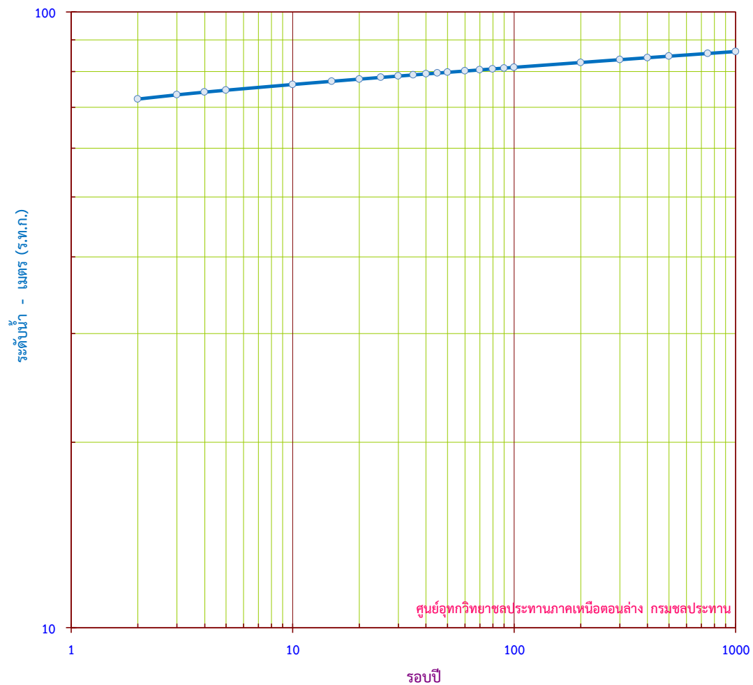
กราฟแสดง ระดับน้ำสูงสุดรายปี ขนาดรอบปีต่างๆ สถานี Y.14 อ.ศรีสีขันาลัย จ.สุโขทัย
