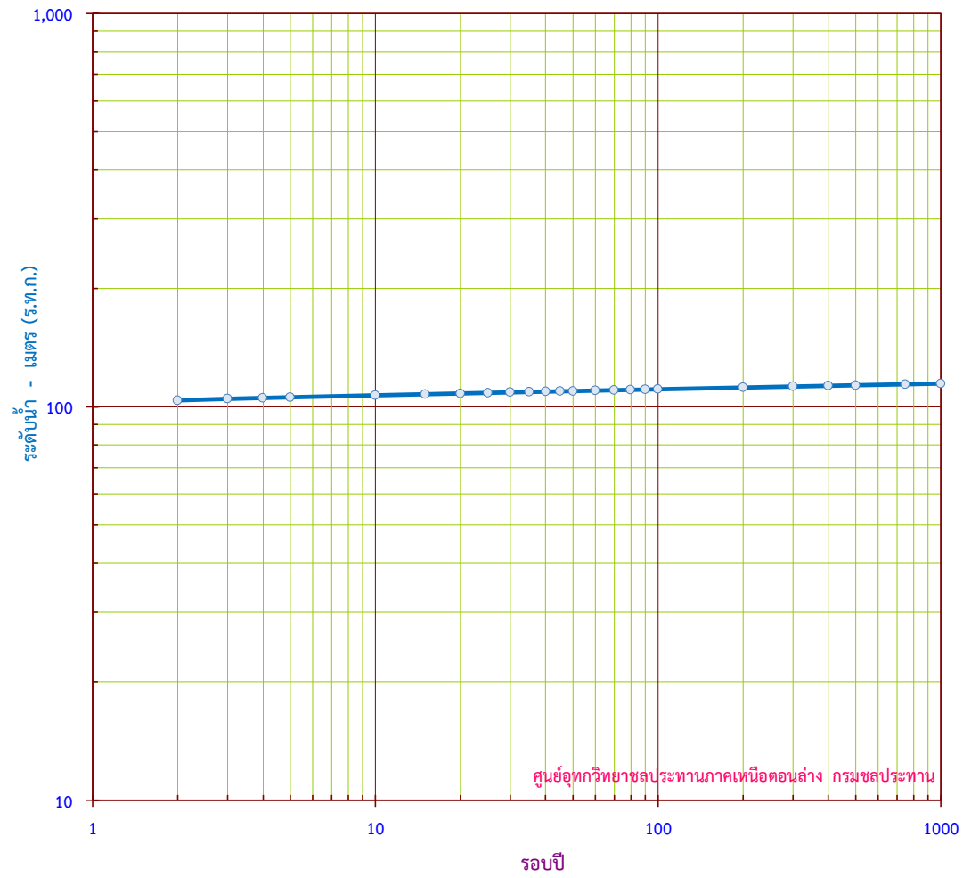
กราฟแสดง ระดับน้ำสูงสุดรายปี ขนาดรอบปีต่างๆ สถานี Y.26 อ.เถิน จ.ลำปาง
