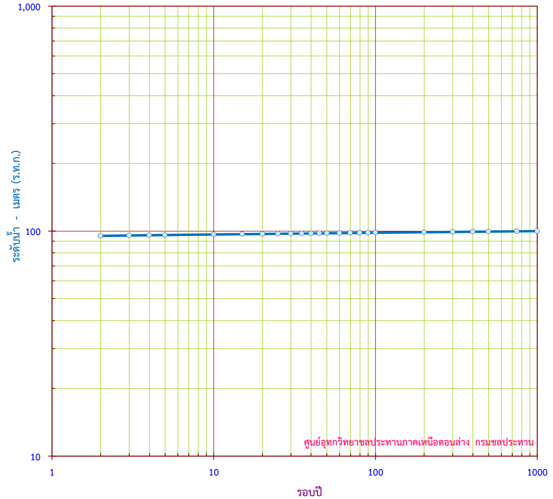
กราฟแสดง ระดับน้ำสูงสุดรายปี ขนาดรอบปีต่างๆ สถานี Y.29อ.ศรีสัชนาลัย จ.สุโขทัย
