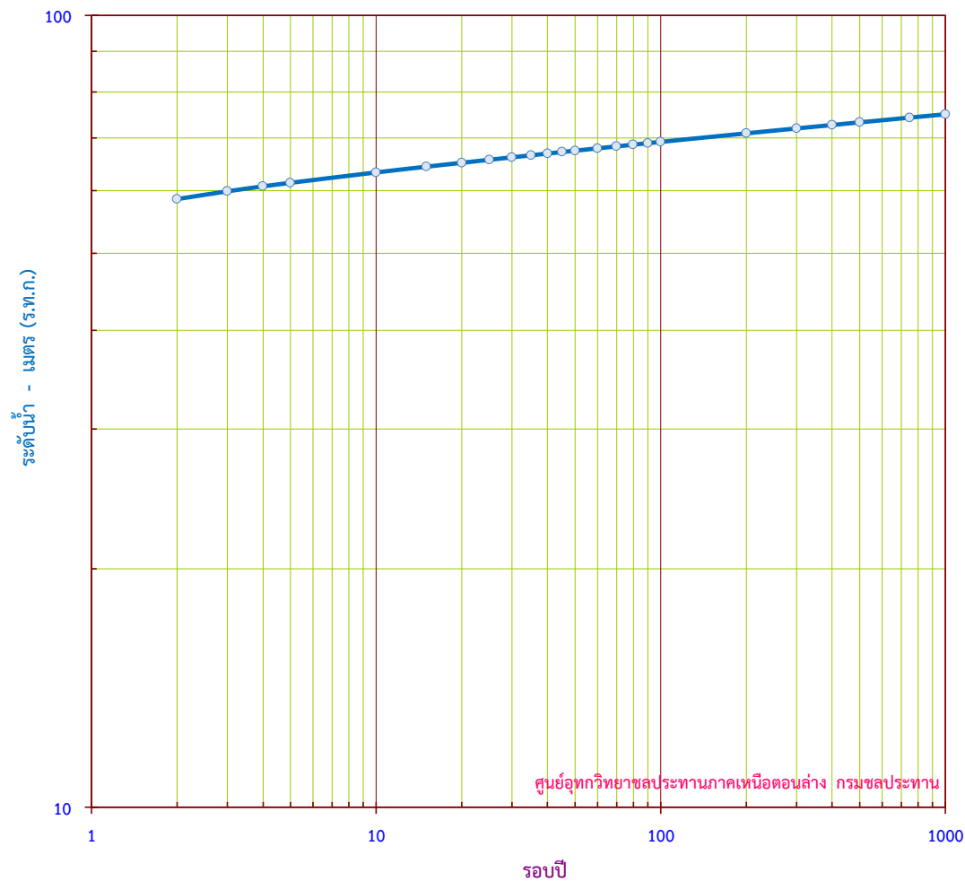
กราฟแสดง ระดับน้ำสูงสุดรายปี ขนาดรอบปีต่างๆ สถานี Y.3A บ.วังขอนไม้ อ.สวรรคโลก จ.สุโขทัย
