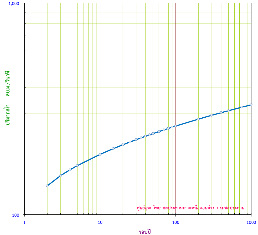
กราฟแสดง ปริมาณน้ำสูงสุดรายปี ขนาดรอบปีต่างๆ สถานี S.4B อ.เมือง จ.เพชรบูรณ์
