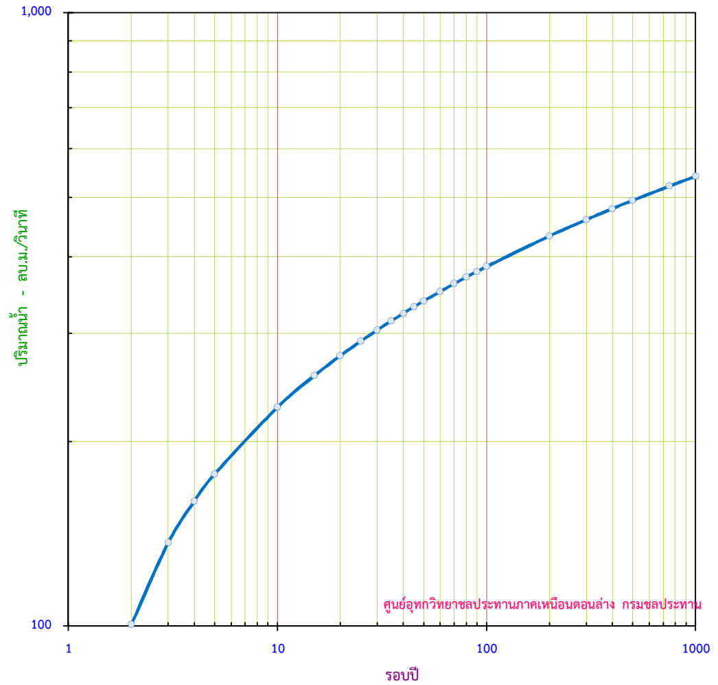
กราฟแสดง ปริมาณน้ำสูงสุดรายปี ขนาดรอบปีต่างๆ สถานี Y.26 อ.เงิน จ.ลำปาง
