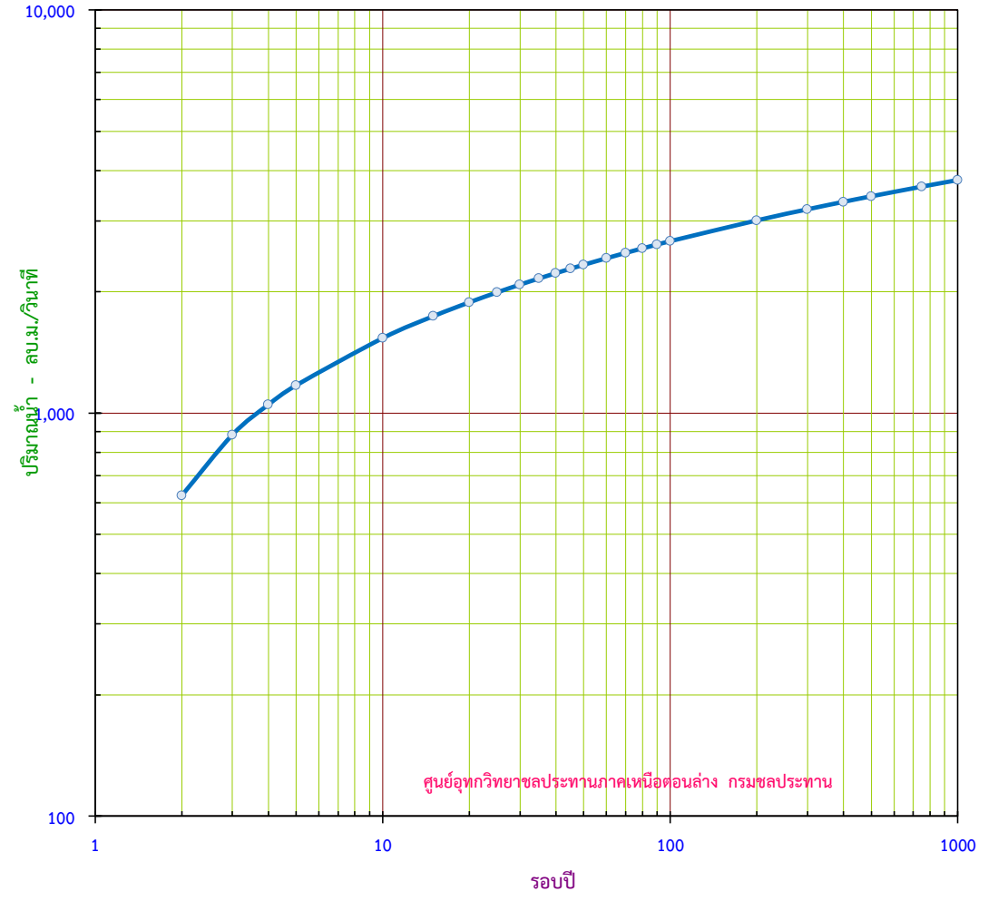
กราฟแสดง ปริมาณน้ำสูงสุดรายปี ขนาดรอบปีต่างๆ สถานี N.12A บ.หาดไผ่ อ.ท่าปลา จ.อุตรดิตถ์
