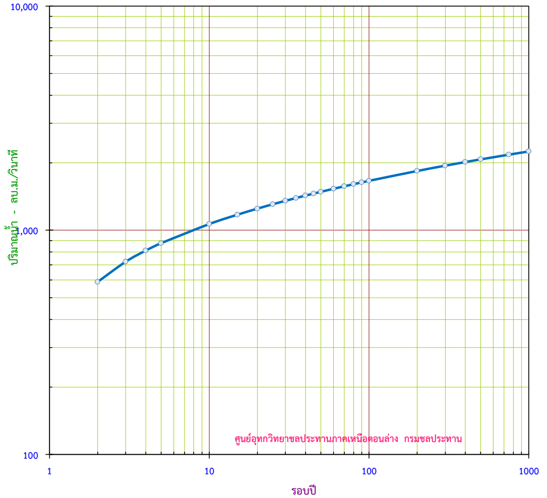
กราฟแสดง ปริมาณน้ำสูงสุดรายปี ขนาดรอบปีต่างๆ สถานี N.27A บ.ท้ายเขื่อนนเรศวร อ.พหลโยธิน จ.พิษณุโลก
