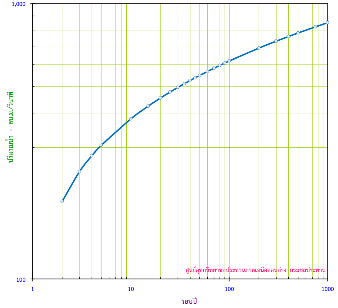
กราฟแสดง ปริมาณน้ำสูงสุดรายปี ขนาดรอบปีต่างๆ สถานี N.36 บ.หนองกระท้าว อ.นครไทย จ.พิษณุโลก
