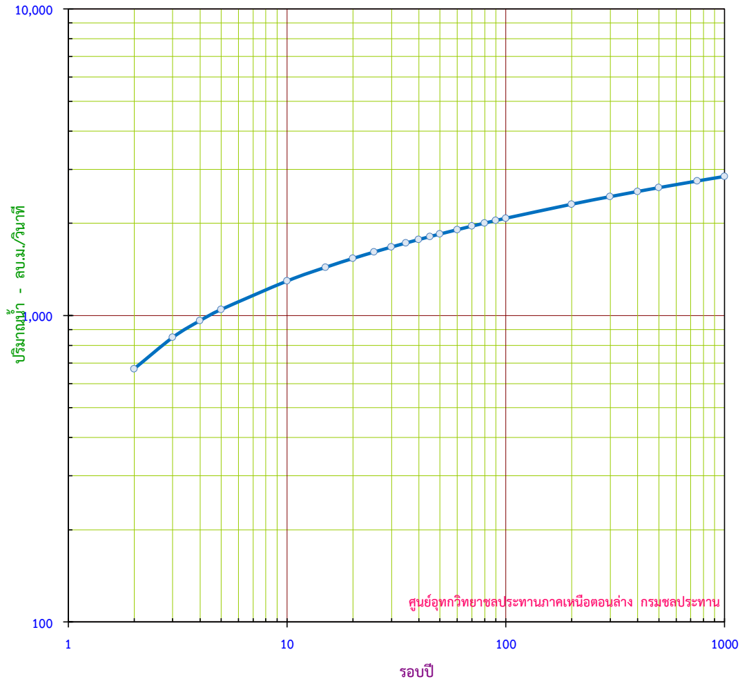
กราฟแสดง ปริมาณน้ำสูงสุดรายปี ขนาดรอบปีต่างๆ สถานี N.60 บ.เด่นลำโรง อ.ตรอน จ.อุดรดิตต์
