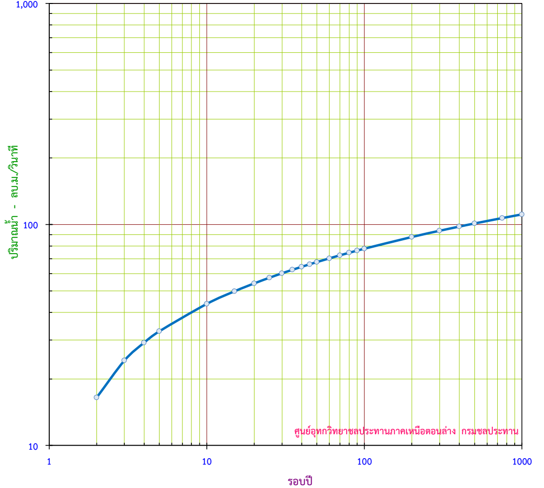
กราฟแสดง ปริมาณน้ำสูงสุดรายปี ขนาดรอบปีต่างๆ สถานี N.82 บ. แก่งทรายงาม อ. ทำปลา จ. อุดรดิษฐ์
