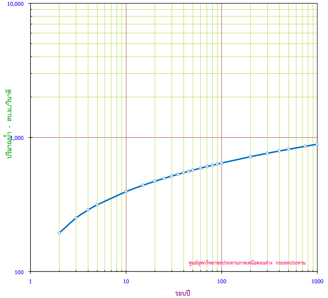
กราฟแสดง ปริมาณน้ำสูงสุดรายปี ขนาดรอบปีต่างๆ สถานี P.26A อ.เมือง จ.กำแพงเพชร
