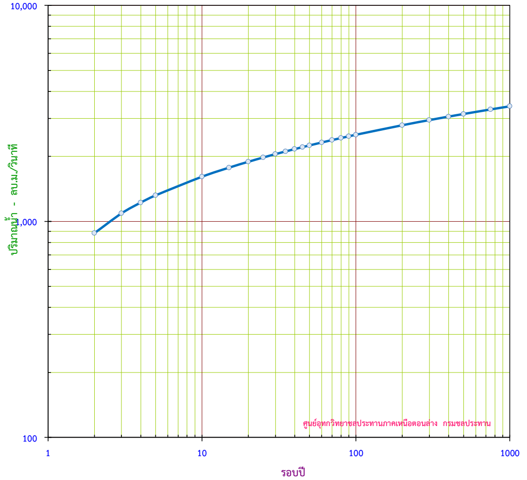
กราฟแสดง ปริมาณน้ำสูงสุดรายปี ขนาดรอบปีต่างๆ สถานี P.7A อ.เมือง จ.กำแพงเพชร
