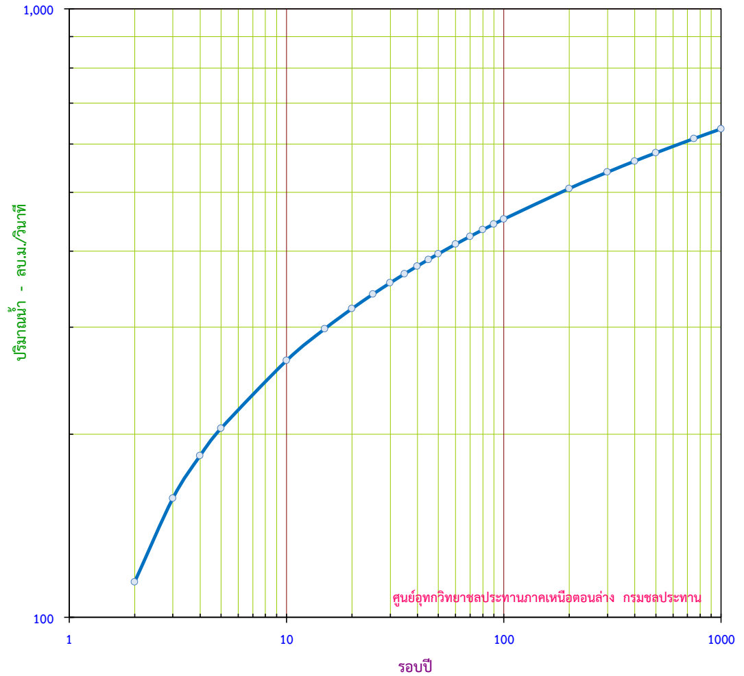
กราฟแสดง ปริมาณน้ำสูงสุดรายปี ขนาดรอบปีต่างๆ สถานี SW.6 อ.แม่สอด จ.ตาก
