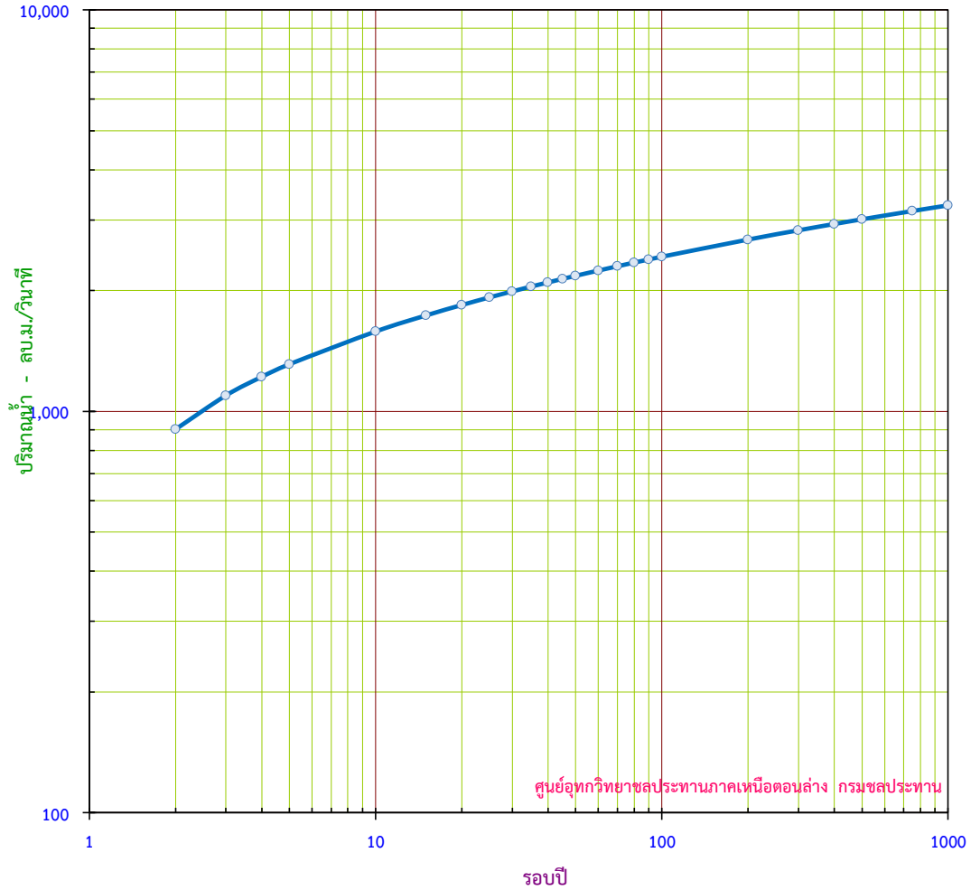
กราฟแสดง ปริมาณน้ำสูงสุดรายปี ขนาดรอบปีต่างๆ สถานี Y.3A บ. วังขอนไม้ อ. สวรรคโลก จ. สุโขทัย
