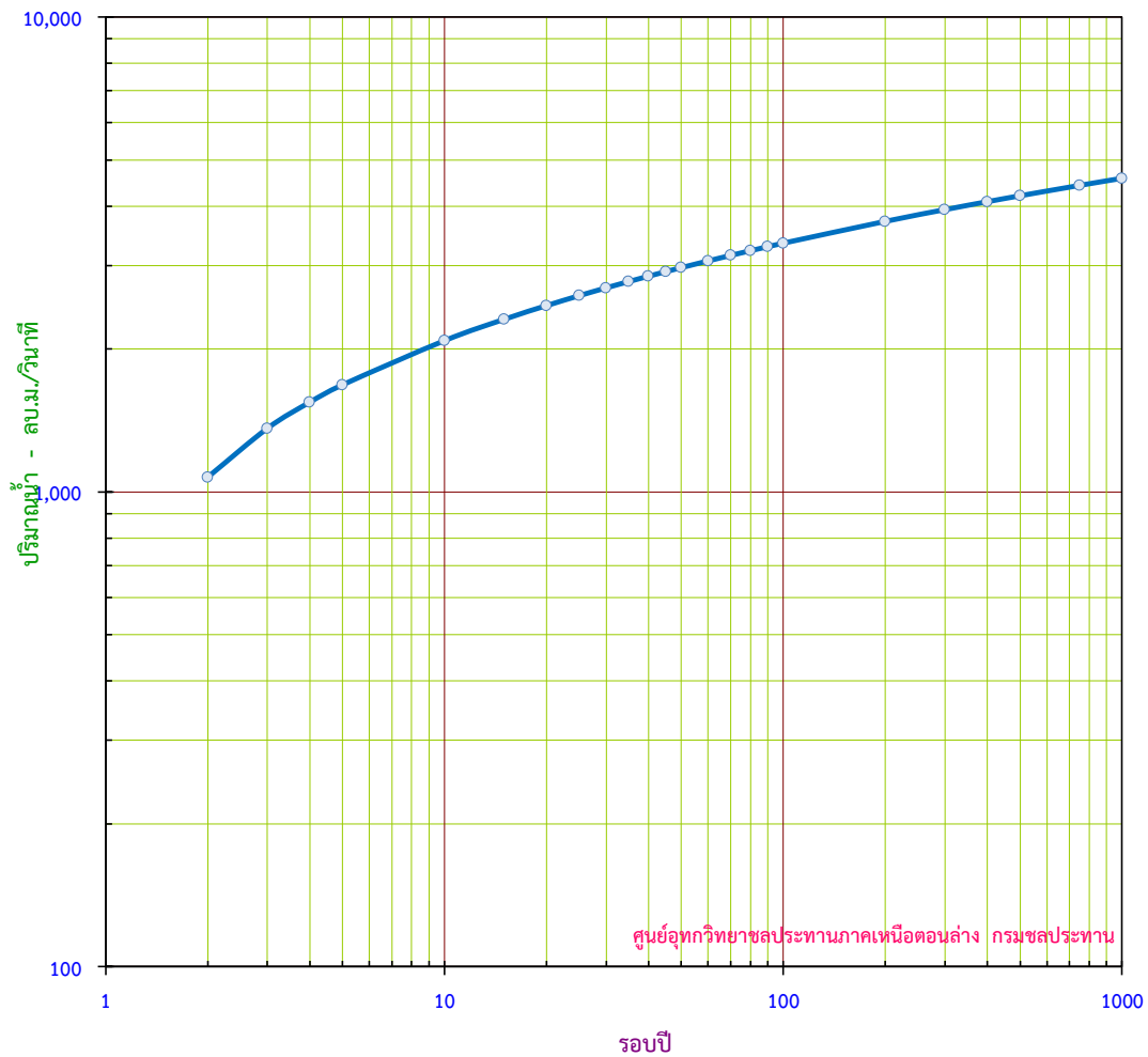
กราฟแสดง ปริมาณน้ำสูงสุดรายปี ขนาดรอบปีต่างๆ สถานี Y.6 บ. แก่งหลวง อ. ศรีสัชนาลัย จ. สุโขทัย
