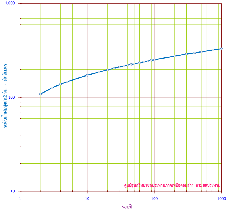
กราฟแสดง ปริมาณน้ำฝนสูงสุด 2 วัน ขนาดรอบปีต่างๆ สถานี 390161 อ.วัดโบสถ์ จ.พิษณุโลก
