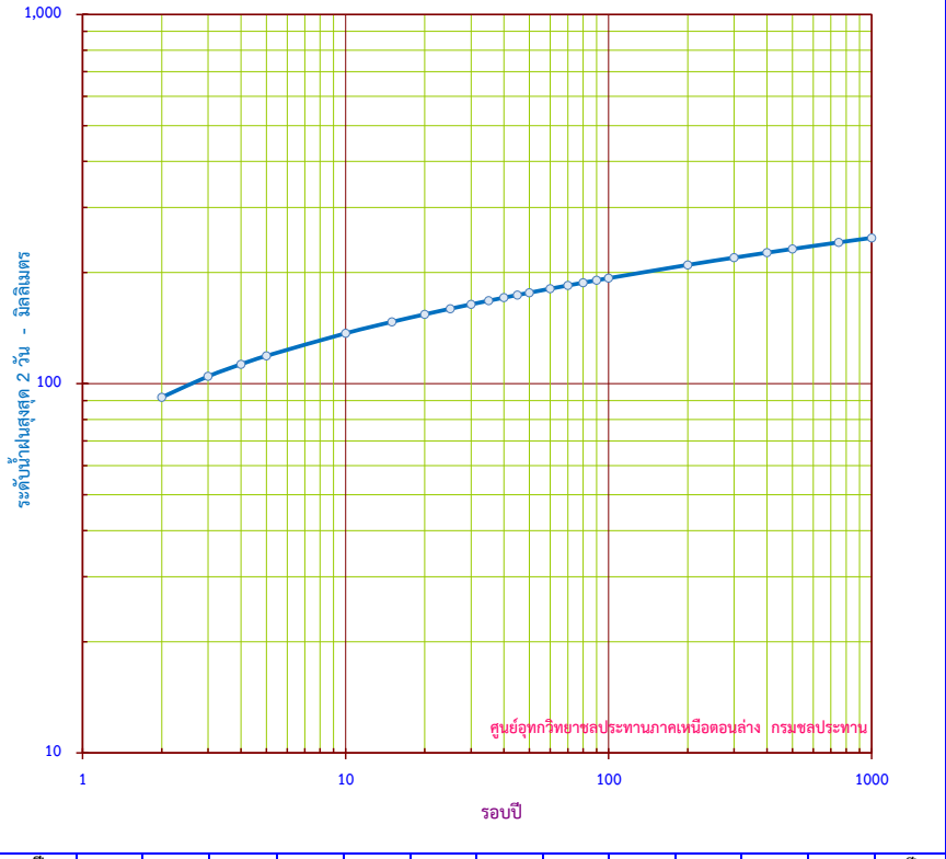
กราฟแสดง ปริมาณน้ำฝนสูงสุด 2 วัน ขนาดรอบปีต่างๆ สถานี 360711 อ.หล่มเก่า จ.เพชรบูรณ์
